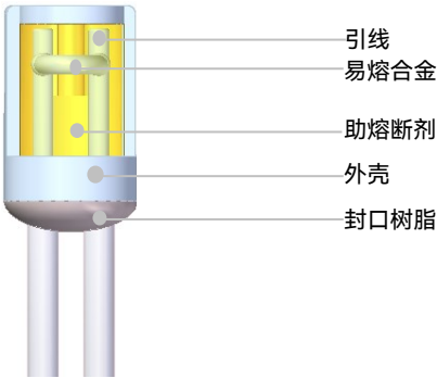
径向型
